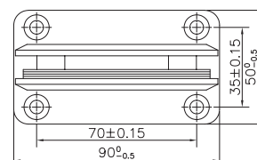
SHH 301 Dimensions
