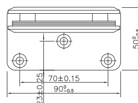
SHH 305 Dimensions
