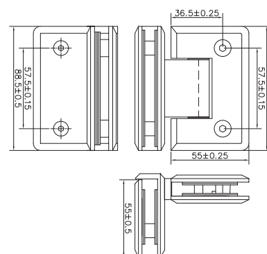
SHH 304 Dimensions
