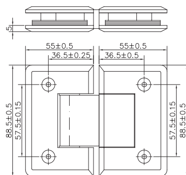
SHH 303 Dimensions
