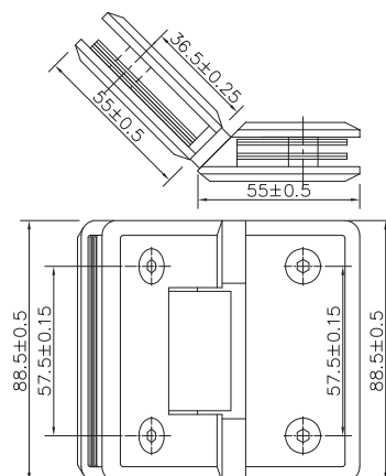
SHH 302 Dimensions
